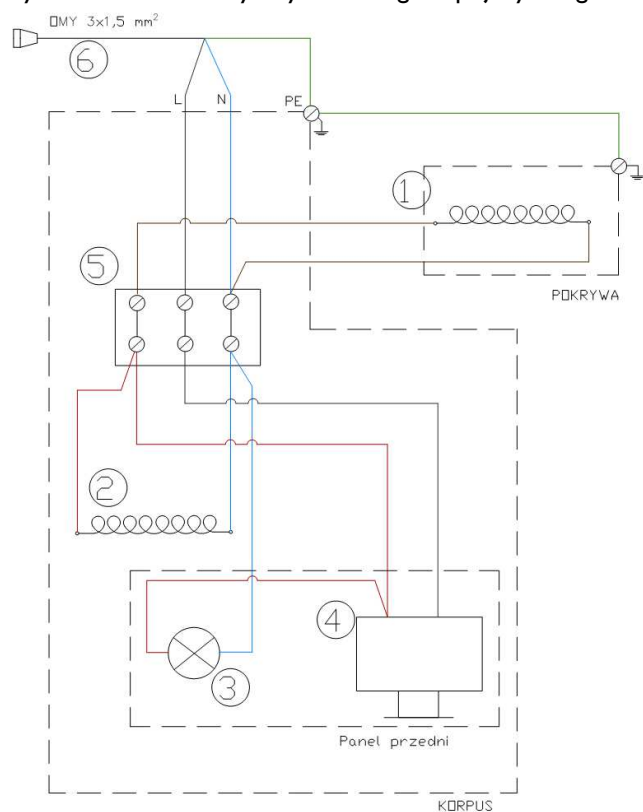
Rys.1. Schemat elektryczny kontakt grilla pojedynczego.
