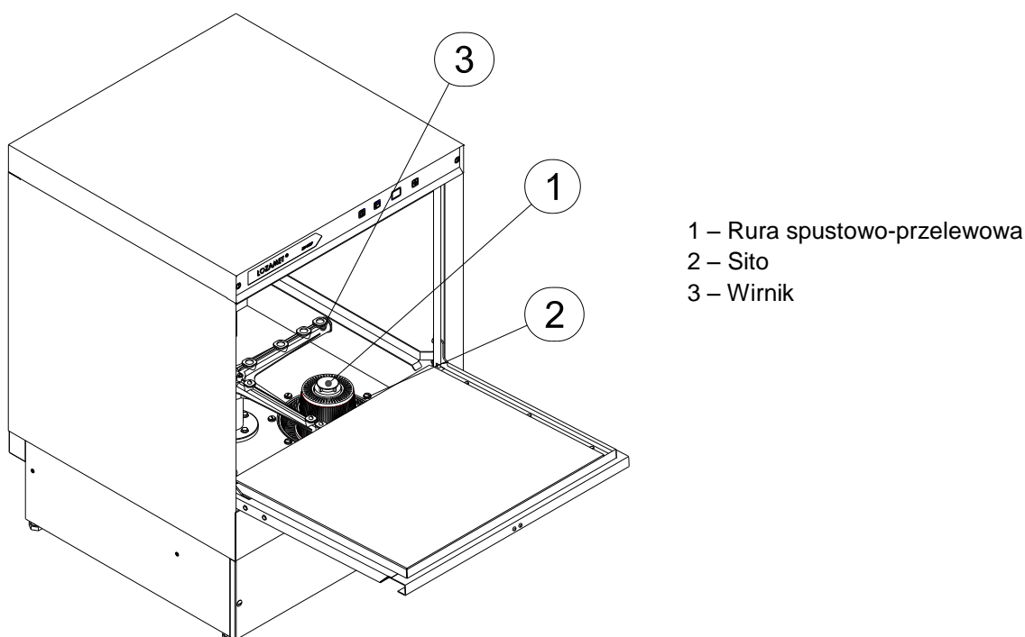
Rys. 6 - Widok komory mycia
