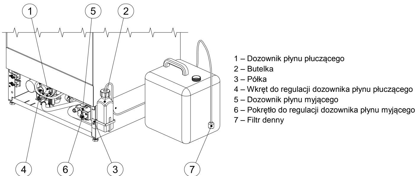
Rys.5 - Podłączenie do zbiorników
