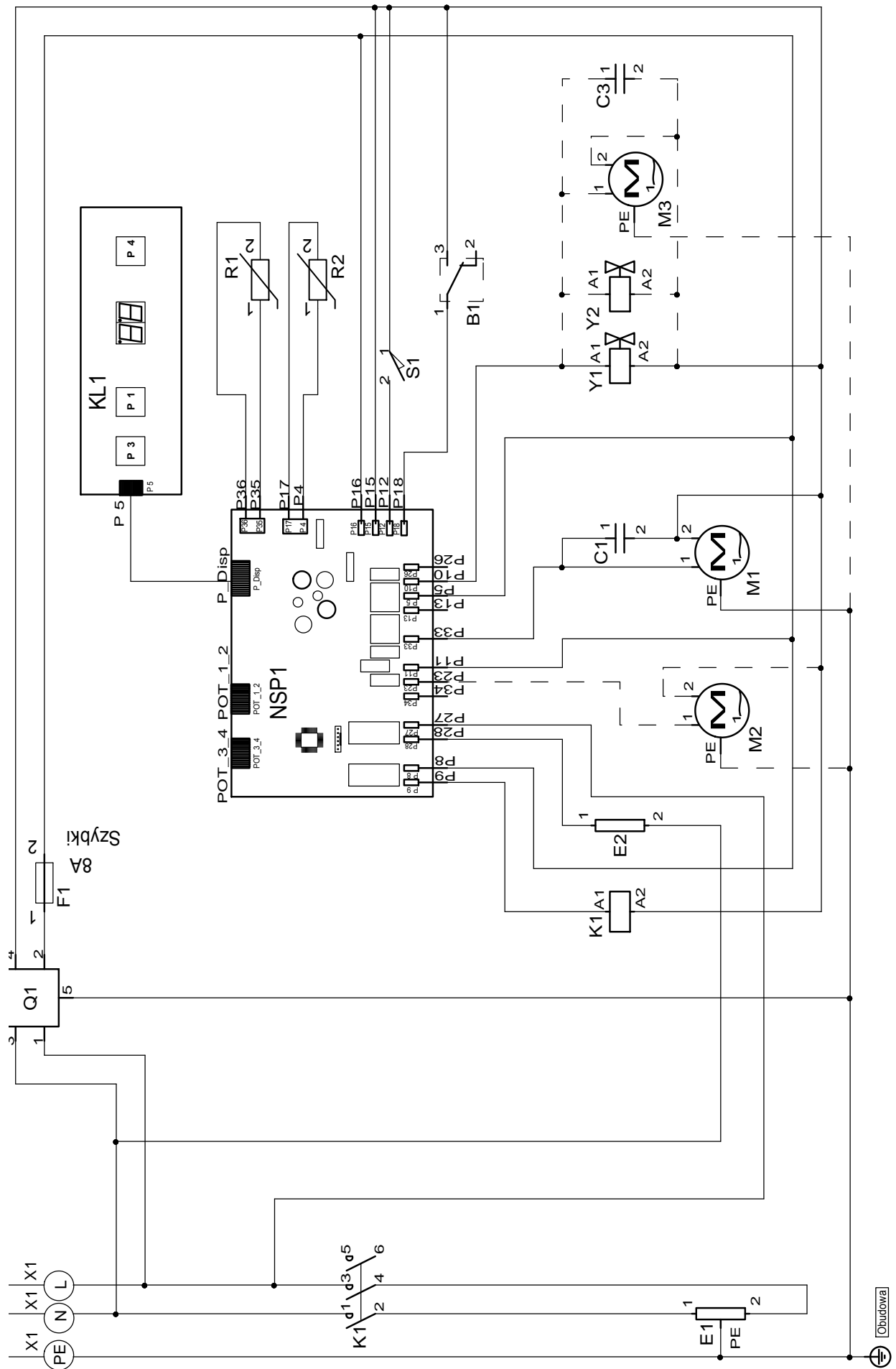
Rys.17 - Schemat instalacji elektrycznej zmywarki ZK-08.4E, ZK-08.4EP
