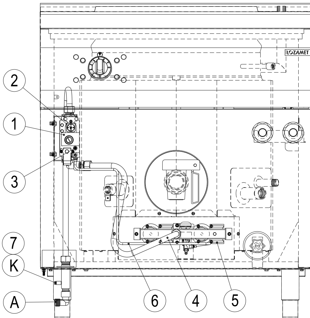
Rysunek 4a - Instalacja gazowa.
