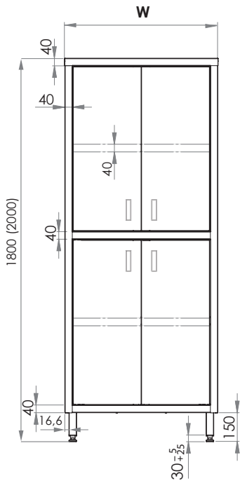
Rzut z przodu
