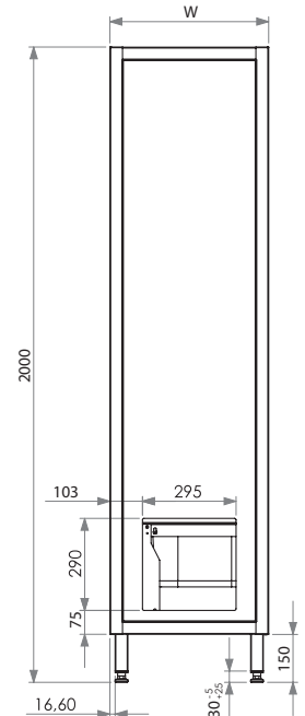
Rzut z tyłu
