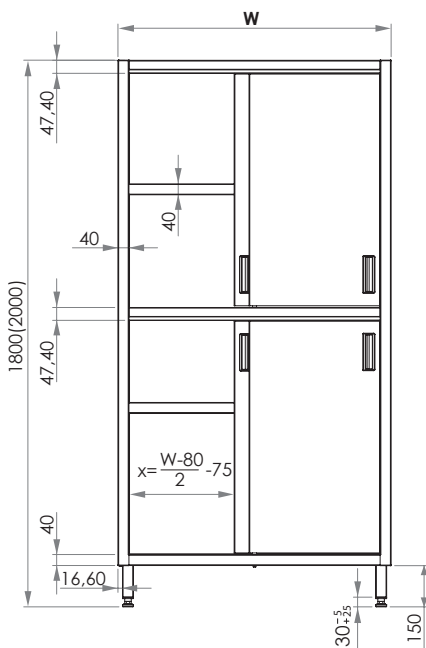
Rzut z przodu
