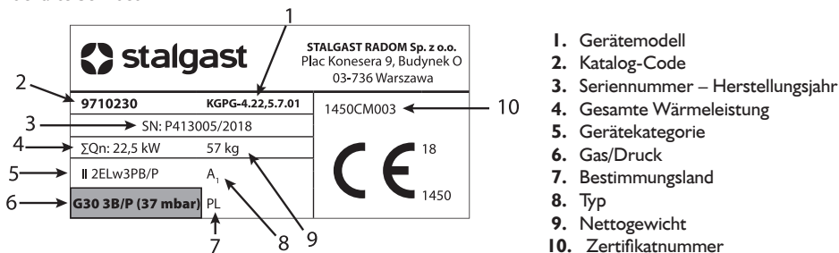
Bild 17. Beispielhaftes Leistungsschild
