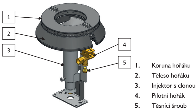
Obrázek 16. Konstrukce hořáku na příkladu 7kW hořáku.
