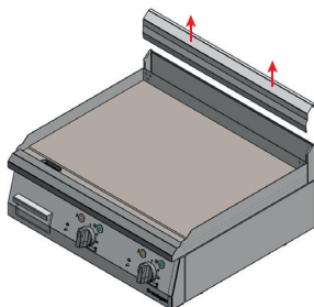
Figura 11. Desmontaje de la tapa de la chimenea.
