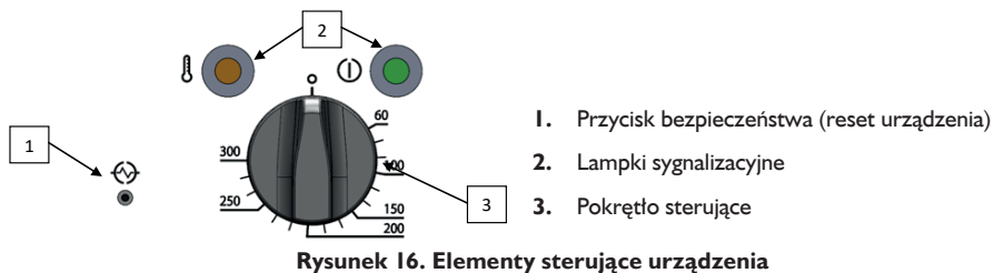
Rysunek 16. Elementy sterujące urządzeniem
