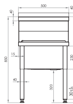
Rzut z przodu
