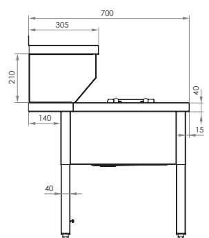
Rzut z boku
