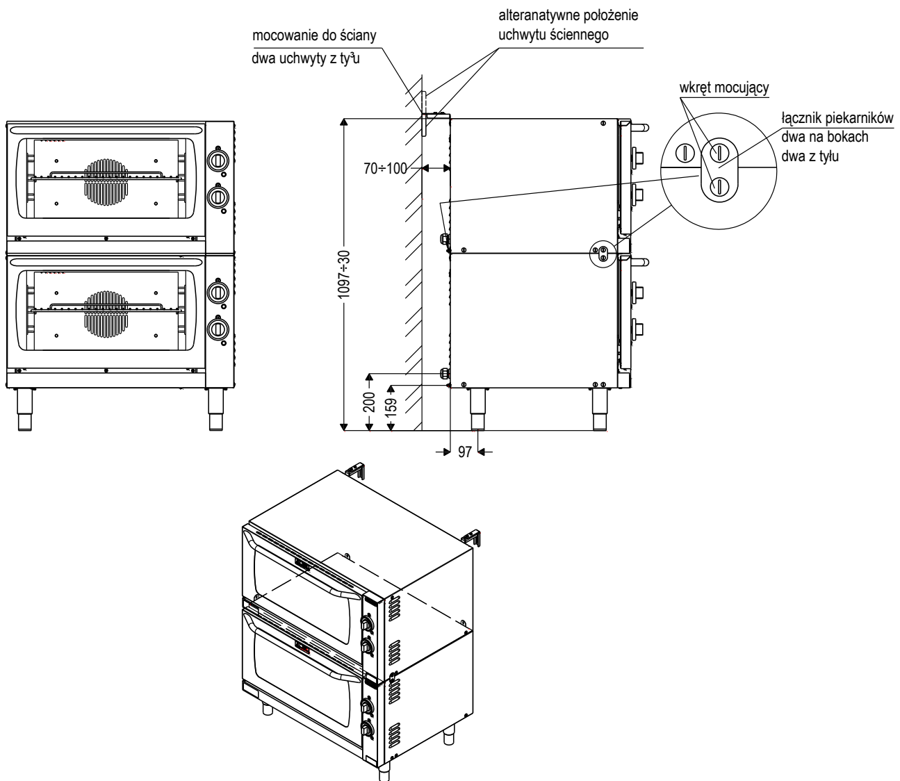
Rysunek 3 - Montaż piekarnika na podstawie
