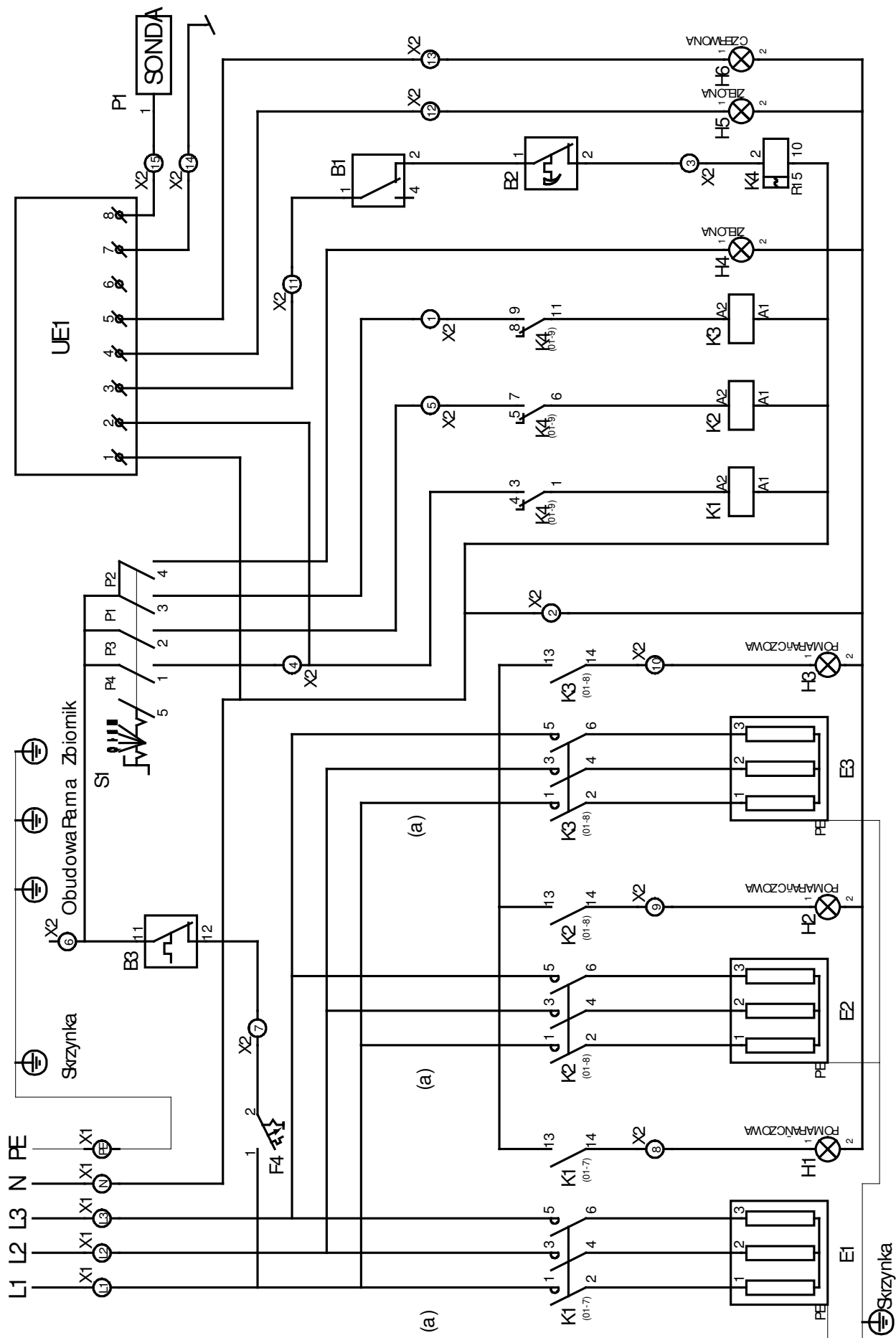
Rysunek 7 – Schemat elektryczny kotłów: WKE- 250.1, WKE- 300.1, WKE-350.1
