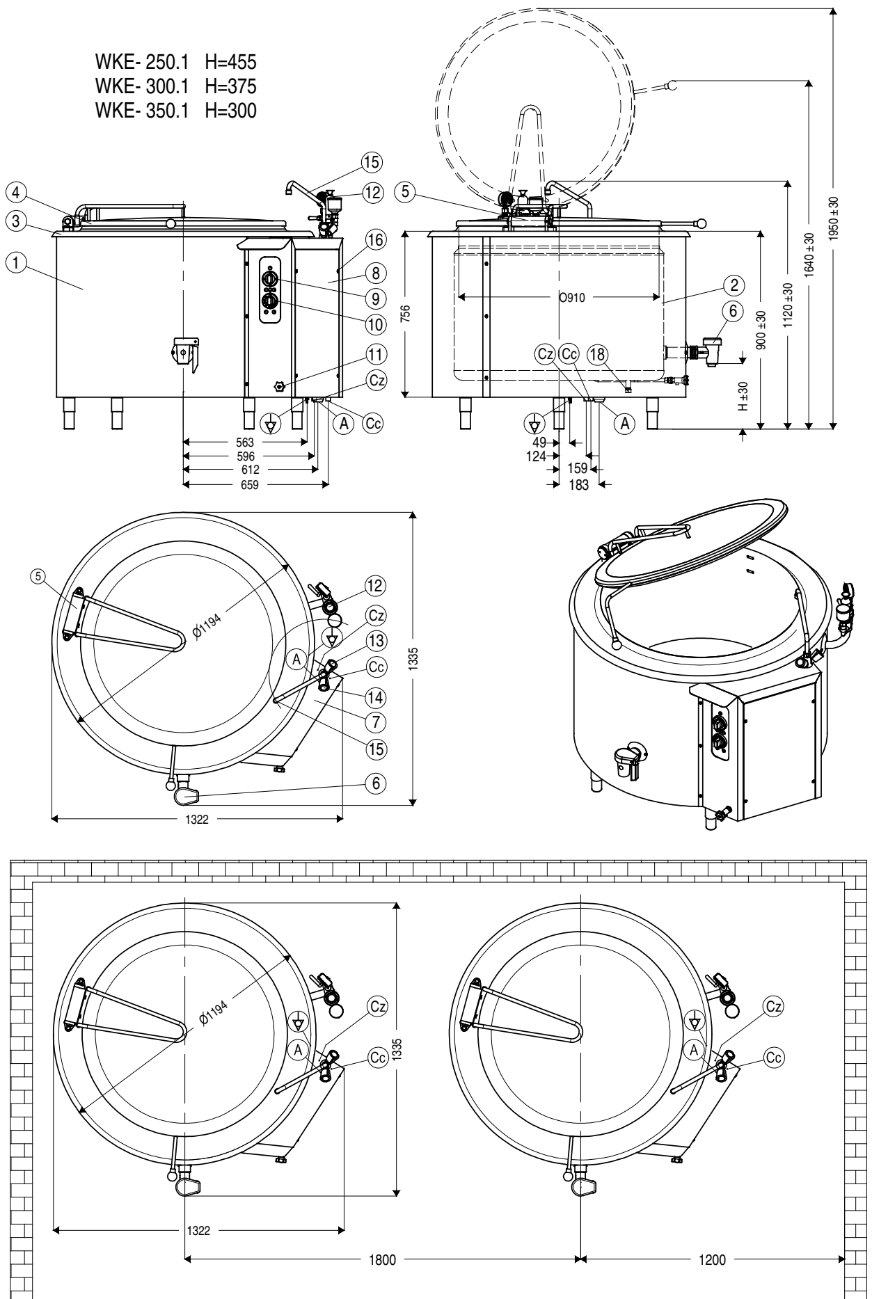
Rysunek 1 - Ogólny widok kotła
