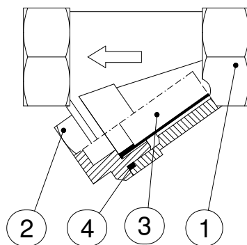
Rys.3 - Osadnik
