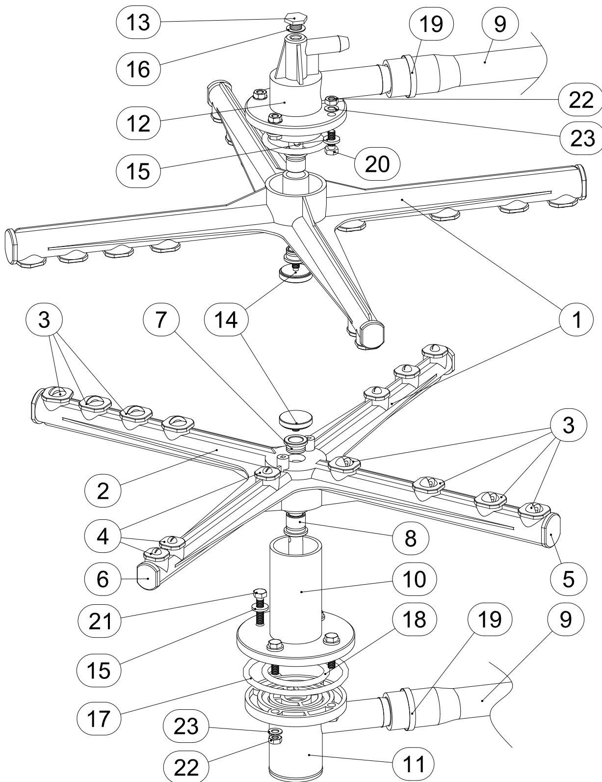
Rys. 16 - Wirniki zmywarki
