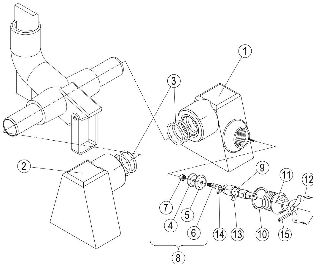
RYSUNEK 5 - Zawór prawy (zasilanie parą) i korpus lewy (odprowadzenie kondensatu)
