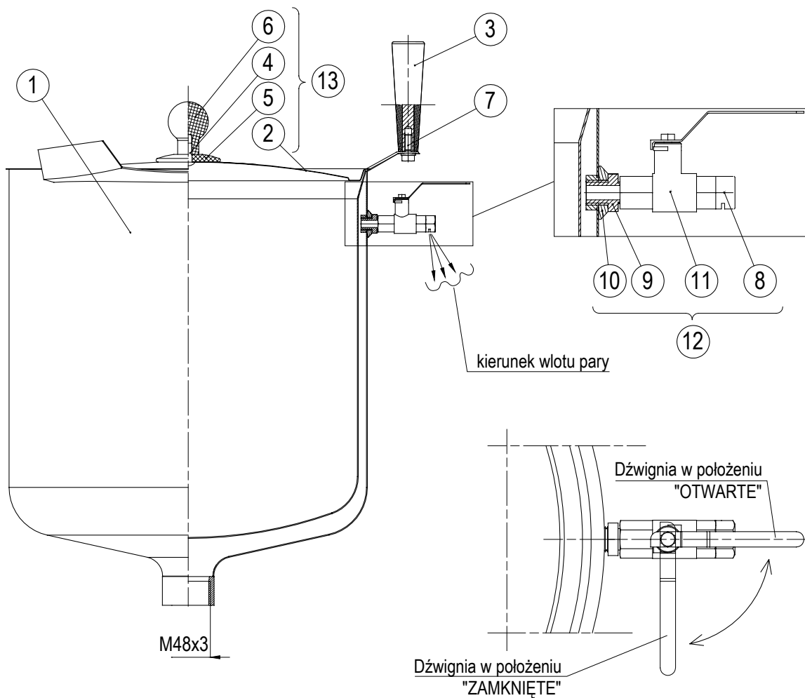
RYСУNEK 3 - Kociołek kompletny
