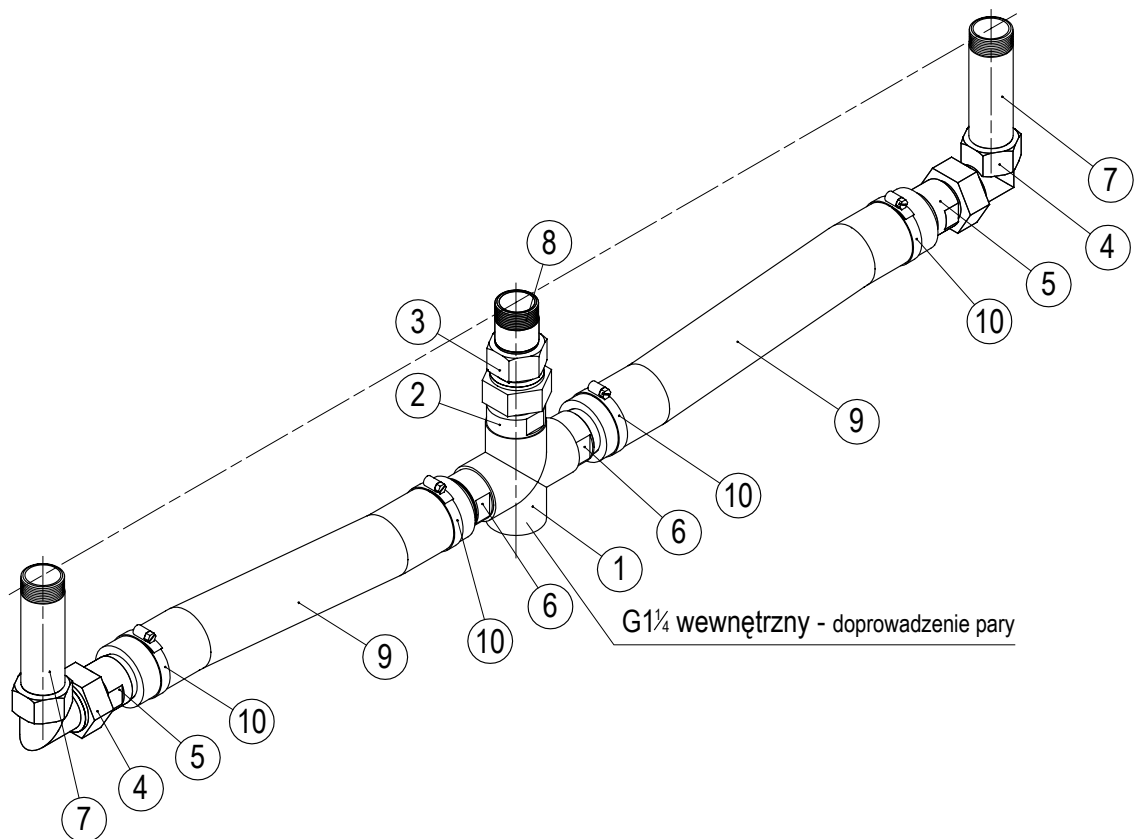
RYSUNEK 7 - Instalacja parowa
