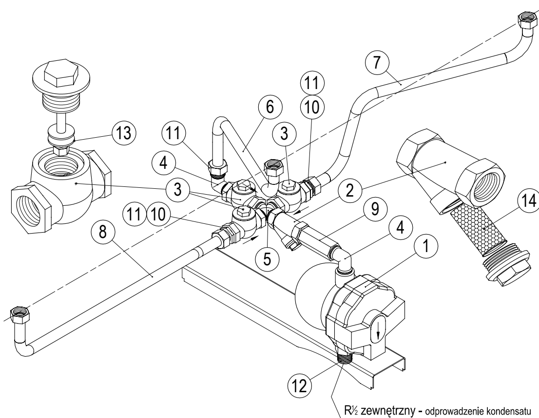
RYSUNEK 6 - Instalacja kondensatu
